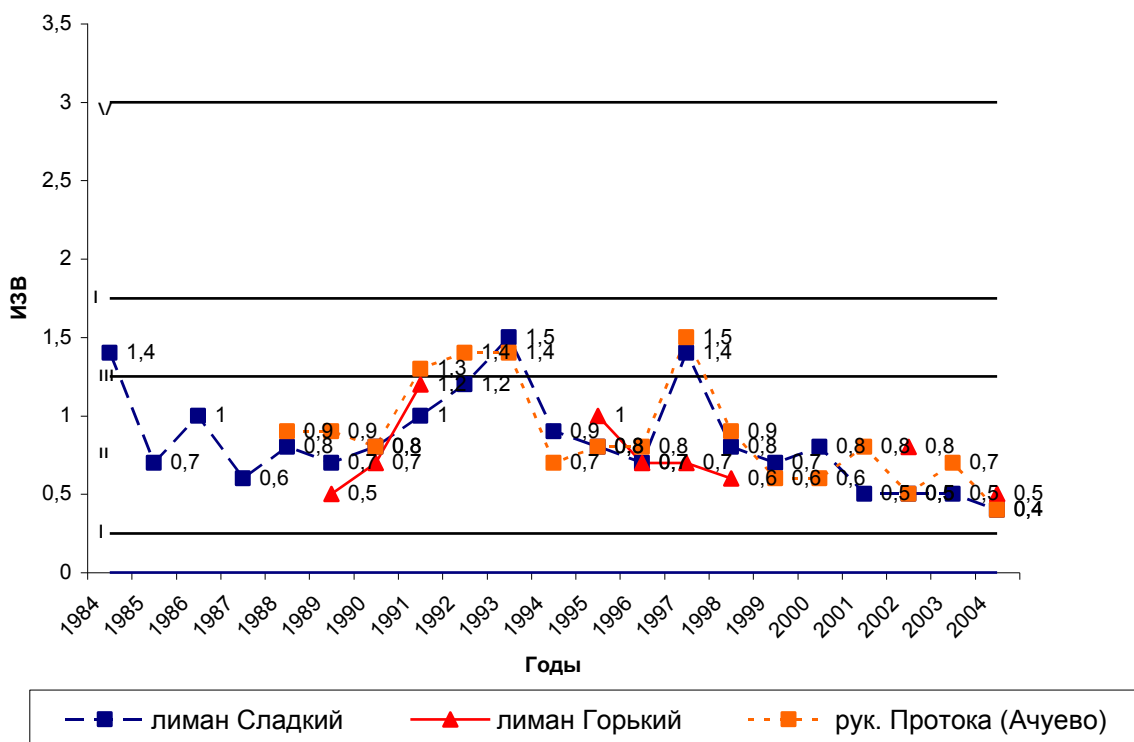
Рис. 3.4. Многолетняя динамика индекса загрязненности вод ИЗВ в водах лиманов Сладкий, Горький и рукава Протока (Ачеуво).
